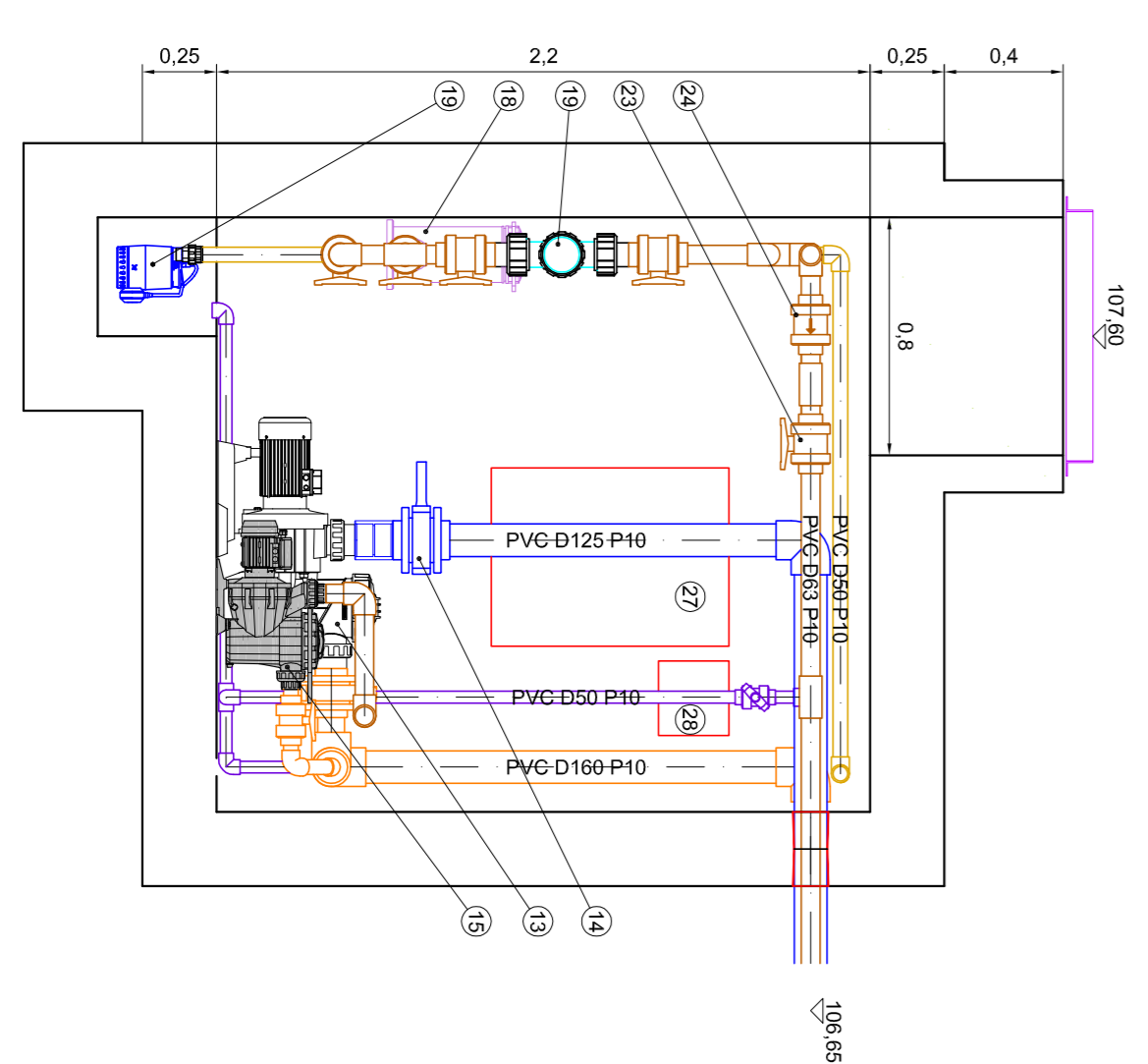
B-B METSZLET
